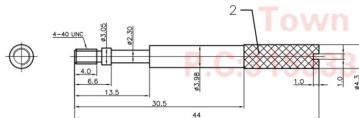
Long BOLT
