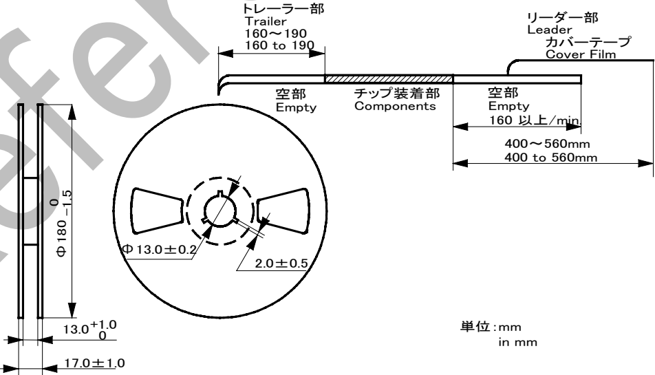
第4図 プラスチックリールの外形寸法図 Figure 4. Dimensions of Plastic Reel (CSTCC3M84G53-R0)
