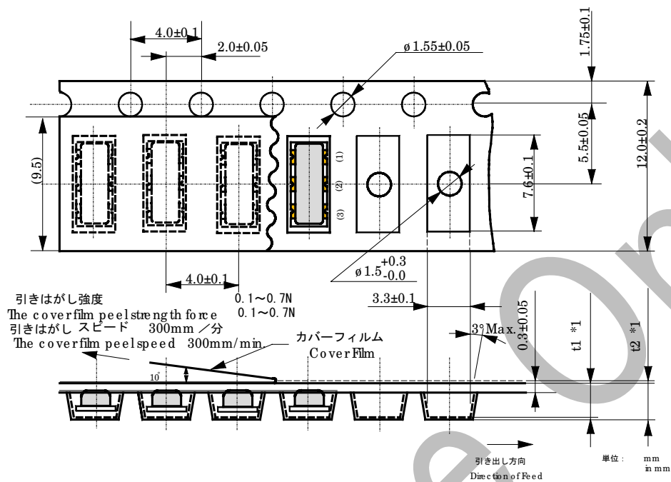
第3図 プラスチックテープの外形寸法図 Figure 3. Dimensions of Plastic Tape (CSTCC3M84G53-R0)
