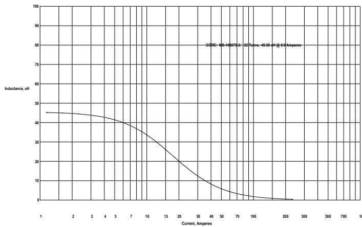
DTMS-27/0,047/15
