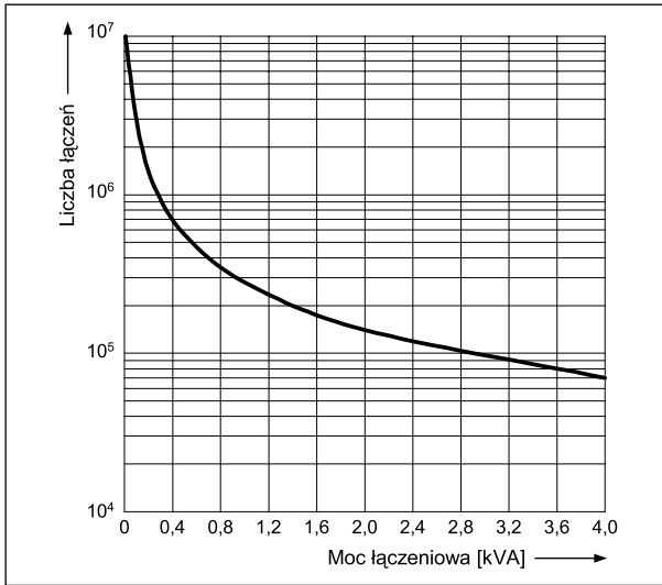
Wykres obciążeń granicznych dla prądu stałego przy obciążeniu rezystancyjnym Wykres 3
