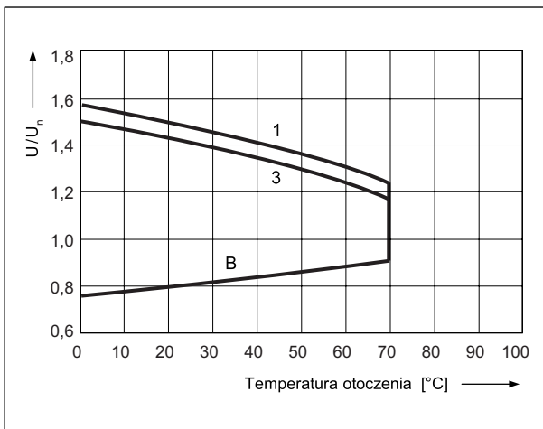
Dopuszczalny zakres napięcia pracy cewki - napięcie zmienne Wykres 5
