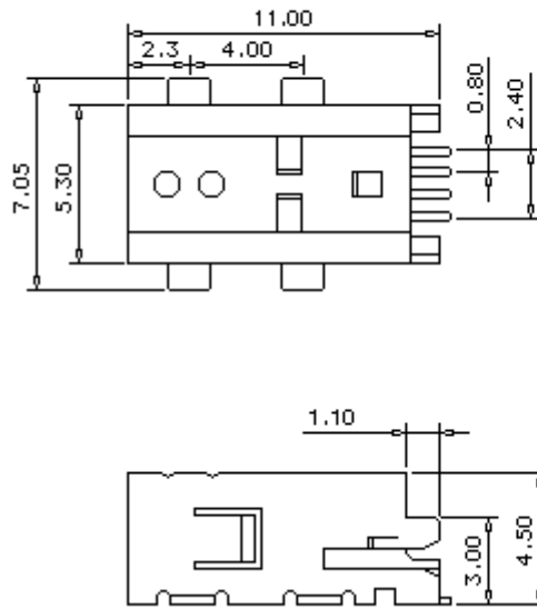
B TYPE CONNECTOR (5 pin) UNIT:mm
