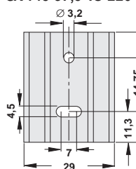
SK 145 37,5 TO 220
