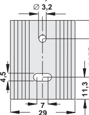
SK 09 37,5 TO 220
