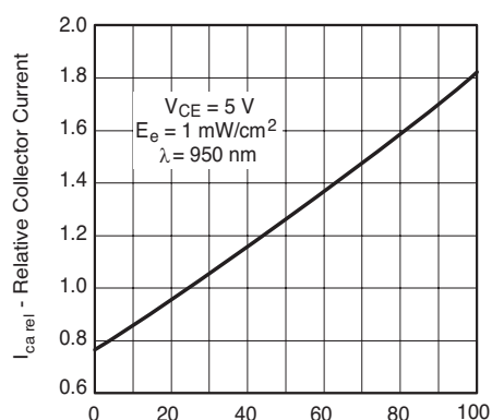
94 8239 T_{amb} - Ambient Temperature (°C)
