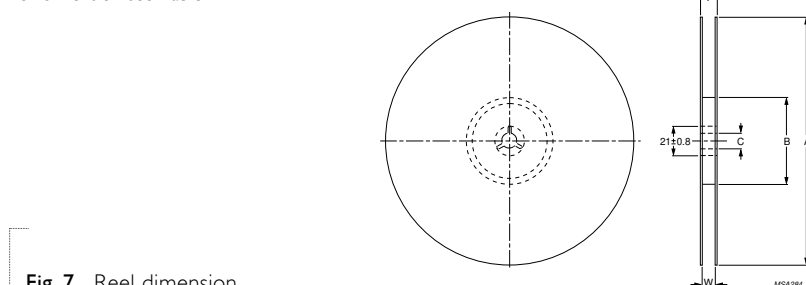
Fig. 7 Reel dimension
