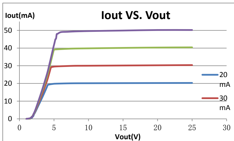
图 2. SM2082ED 恒流曲线图
