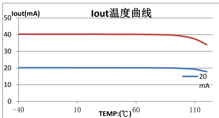
图 3. SM2082ED 输出电流温度特性 ( I_{OUT} = 20mA ; I_{OUT} = 40mA )
