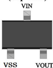
662K./65K5.引脚图
