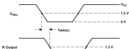
图 7 t_{(WAKE)} 测试电路与电压波形
