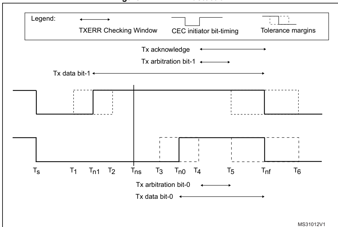
Figure 442. TXERR detection
