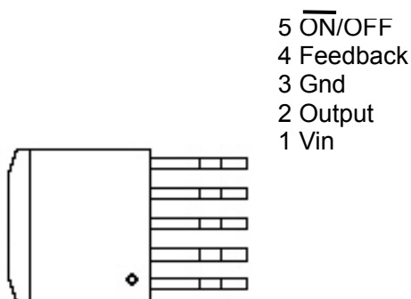
TO220B-5L/TO220-5L
