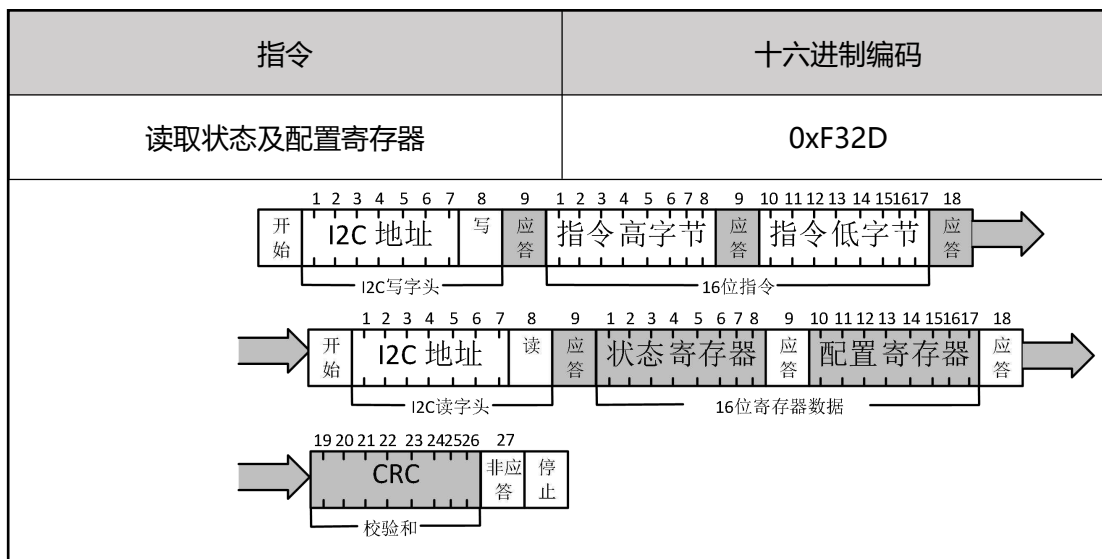
图 10.3-4 读取状态寄存器及配置寄存器指令(白色块由微控制器控制，传感器响应为灰色块)
