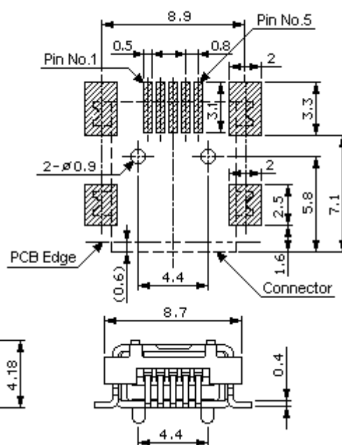
P.C.B. LAYOUT
