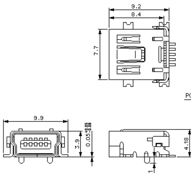
B TYPE CONNECTOR (5 pin) UNIT:mm
