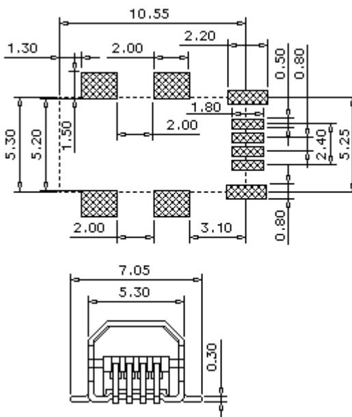
P.C.B. LAYOUT
