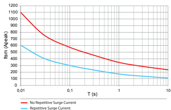
GN - 125 A
