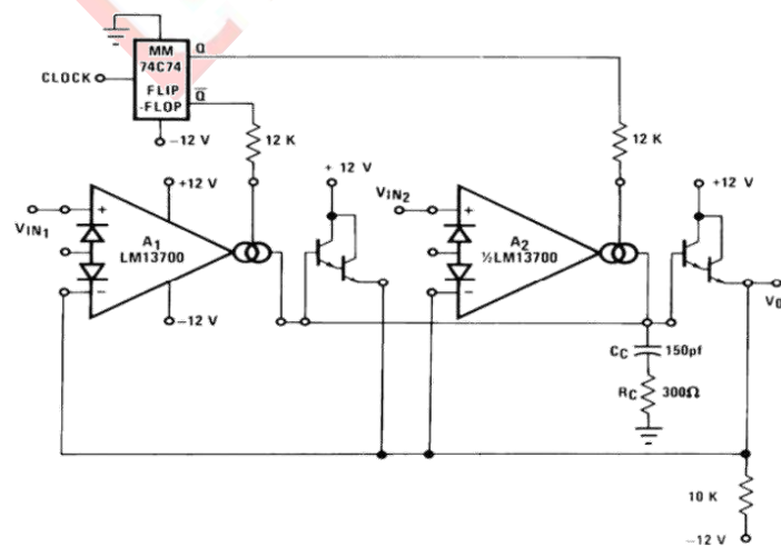
图 19 多路复用器
