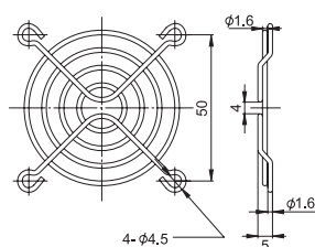
FG-06 For 60mm Fan
