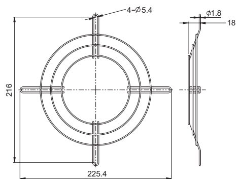
FG-18B For 176mm Fan
