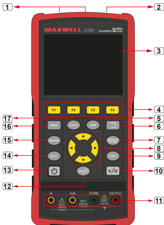
Panoul frontal al osciloscopului
