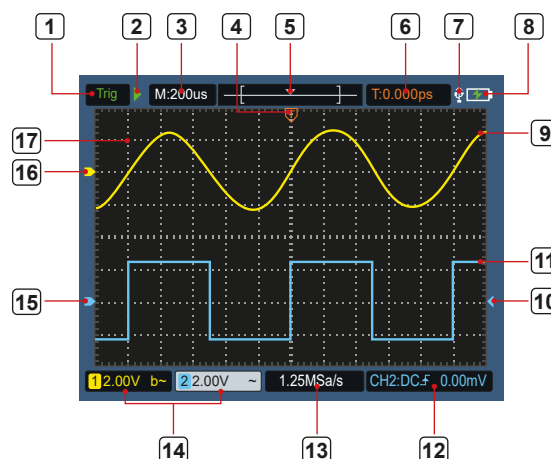
5. obraz : Uživatelské rozhraní osciloskopu
