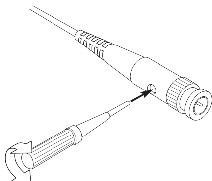
0-3. Obrázok: Nastavenie sondy
