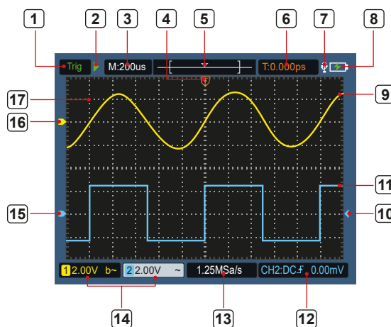
Figura 5: Interfața cu utilizatorul osciloscopului
