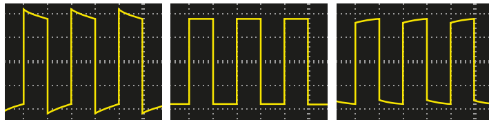
0-2. Figura: Afișarea formei de undă de compensare a sondei
