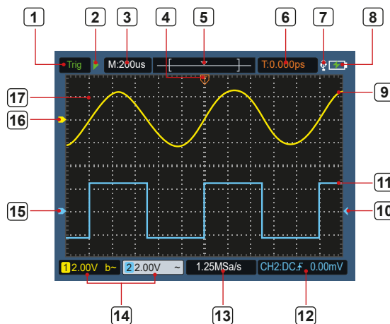
5. ábra: Az oszcilloszkóp felhasználói felülete
