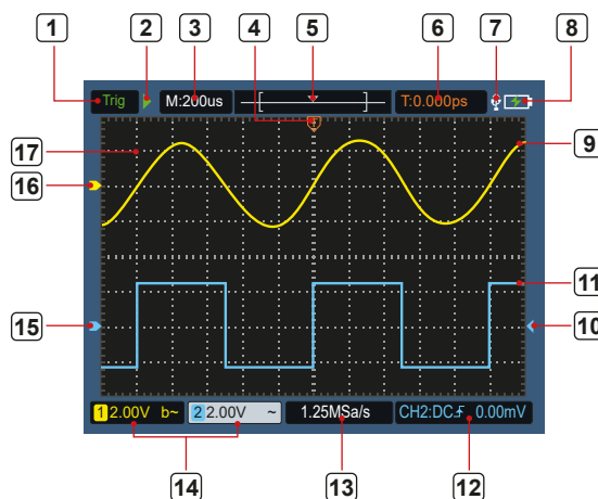
5. obraz: Používateľské rozhranie osciloskopu
