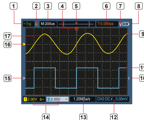
Abbildung 5: Benutzeroberfläche des Oszilloskops
