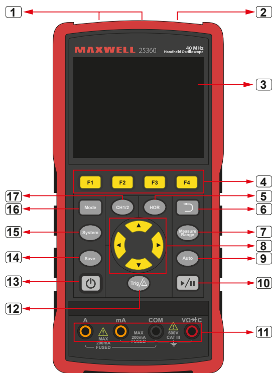
Predný panel osciloskopu
