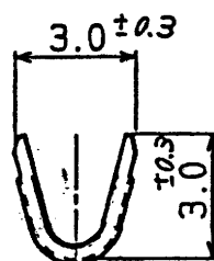
A-A SEC.
