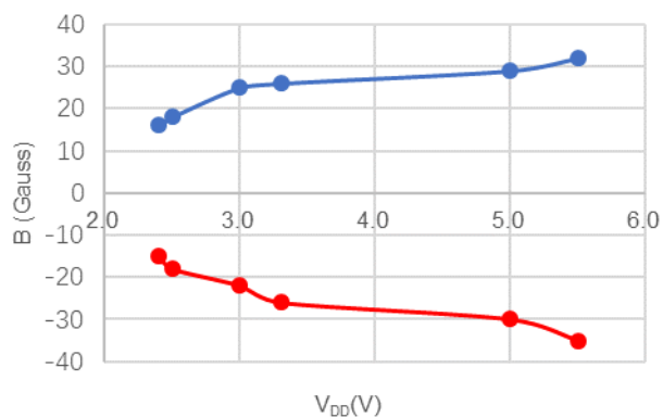
磁感应点 vs. 工作电压
