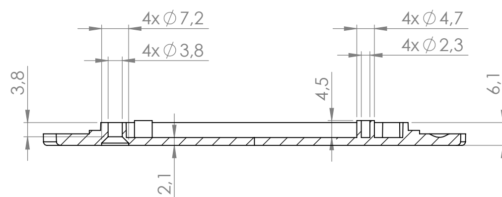
SECTION D-D
