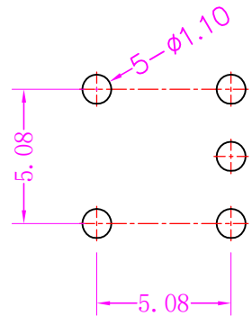
安装孔尺寸
