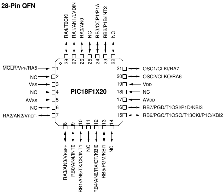
28-Pin QFN
