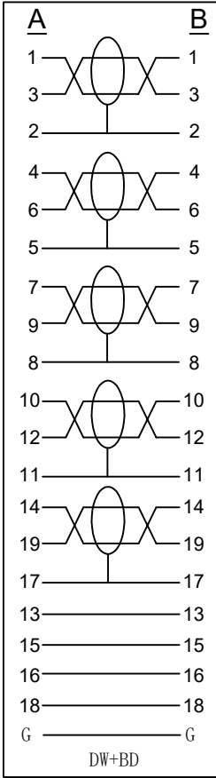
WIRING DIAGRAM:
