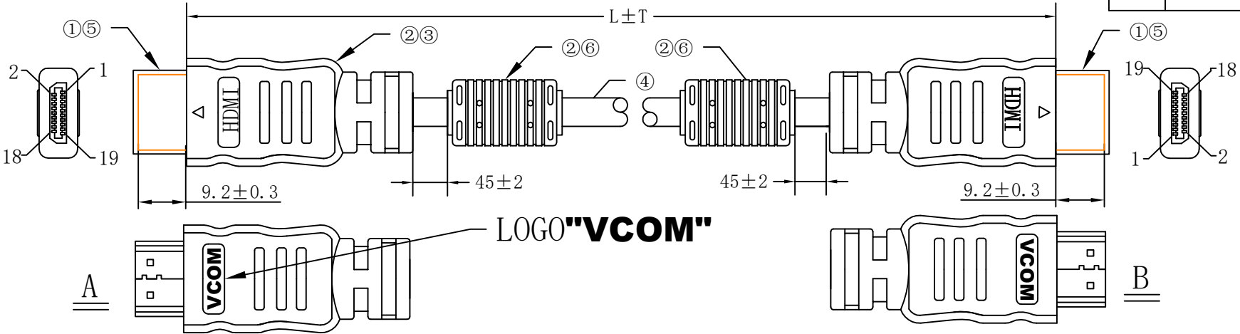
WIRING DIAGRAM:
