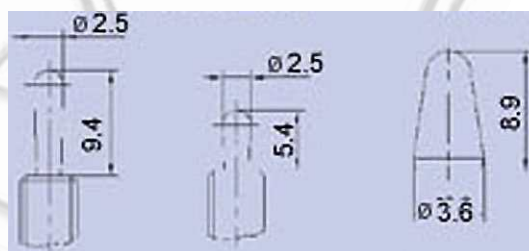
Standard (A) Short (C) Toggle (D)
