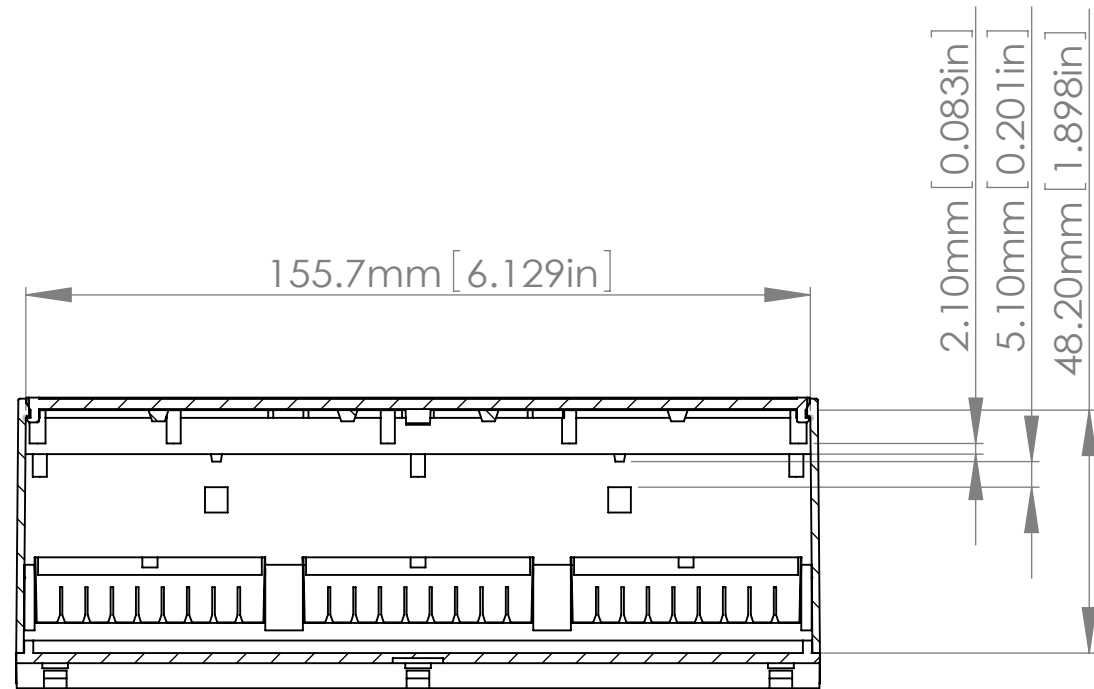
SECTION A-A SCALE 2 : 3
